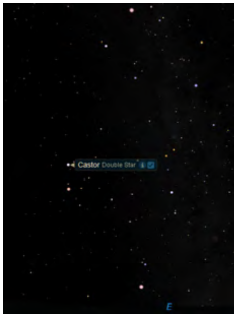
Fig. 5 Tvillingerne med Castor og dens tvilling Pollux lige syd for. Konfiguration den 15. december 2017, set fra sydfyn kl. 20:00. Castor ses i østnordøstlig retning 24 grader over horisonten. Klokket 22:00 i stik østlig retning. Mælkevejen anes lige til højre for Tvillingerne. Allerøverst ses en tydelig (dobbel)stjerne Capella i stjernebilledet Kusken (Auriga).
