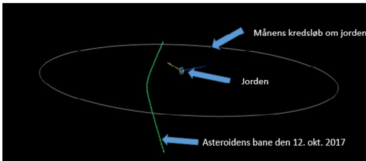
Fig. 1 Asteroiden 2012 TC4's bane den 12. oktober 2017
