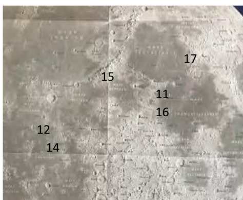
Placeringen af Apollo 11, 12, 14, 15, 16 og 17's bemandede månelandinger
