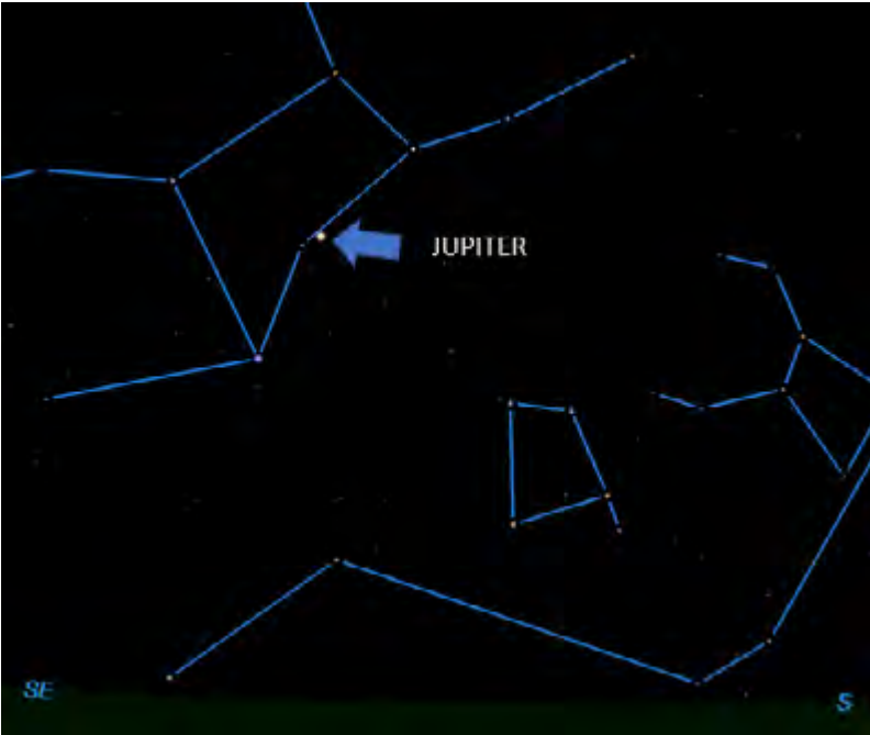
Figur 1: Planeten Jupiter i stjernetegnet JOMFRUEN 14. april 2017 kl. 22:00, ca. 27 grader over horisonten i retning mellem sydøst og syd. Ved midnat står Jupiter i stik syd denne aften.
