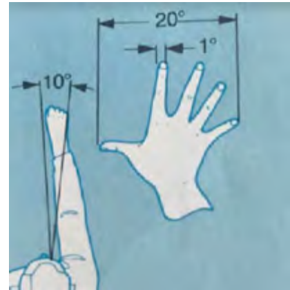
Figur 2: Vinkelmåling ved udstrakt arm: Pegefingeren = 1 grad, Håndsbredde=10 grader, Udstrakt hånd=20 grader
