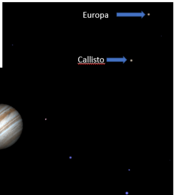
Figur 3: Jupiter med de inderste 4 måner: Io, Europa, Ganymede og Callisto som de ser ud den 14. april 2017 kl. 22:00.
