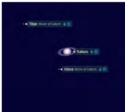
Fig. 2: Saturn med månerne Titan og Rhea kl 0100, den 28. juni 2018. Cassini Devisjonen, der deler ringene kan lige anes på billedet. Bemærk at Titan flytter sig relativt hurtigt, idet den er 16 døgn om at flyve rundt om Saturn.
