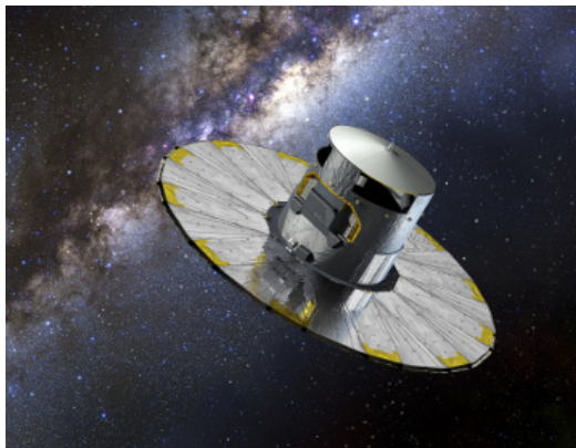
Fig.3 GAIA rumsonden opsendt i 2013 og placeret i den stationære såkaldte L2 position hvor jorden skygger for solen. (L2: Lagrange 2 punktet)
